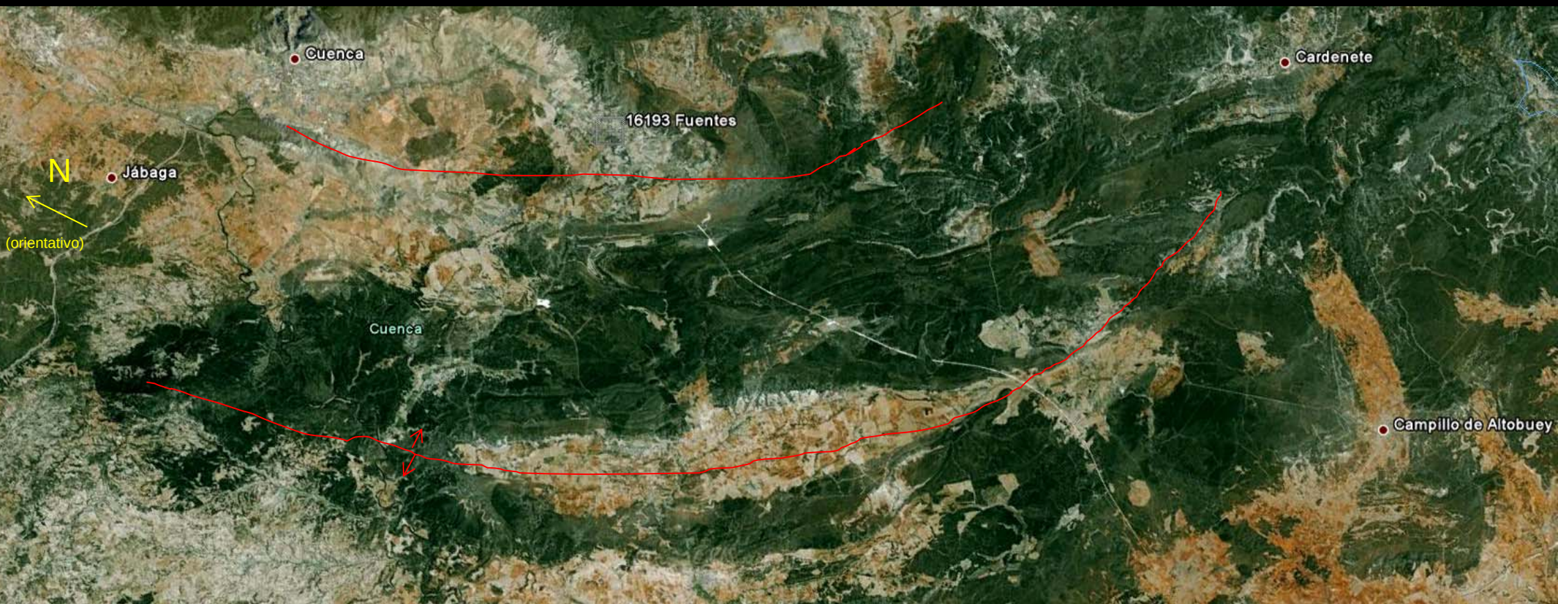
Las largas estructuras anticlinales y sinclinales de las Hojas de Fuentes y Valera de Abajo.
