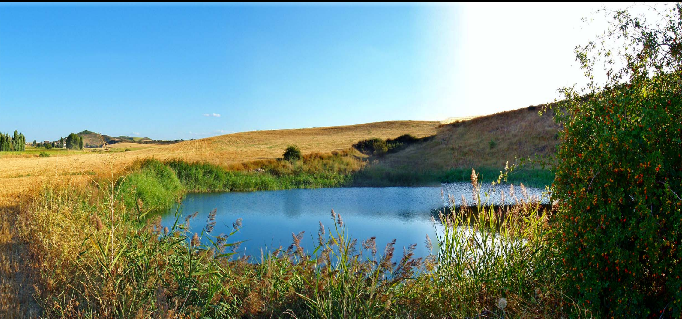
Laguna Ojo de La Corva. N de Fuentes. N Centro Hoja de Fuentes. (por Javibancero-Google)
